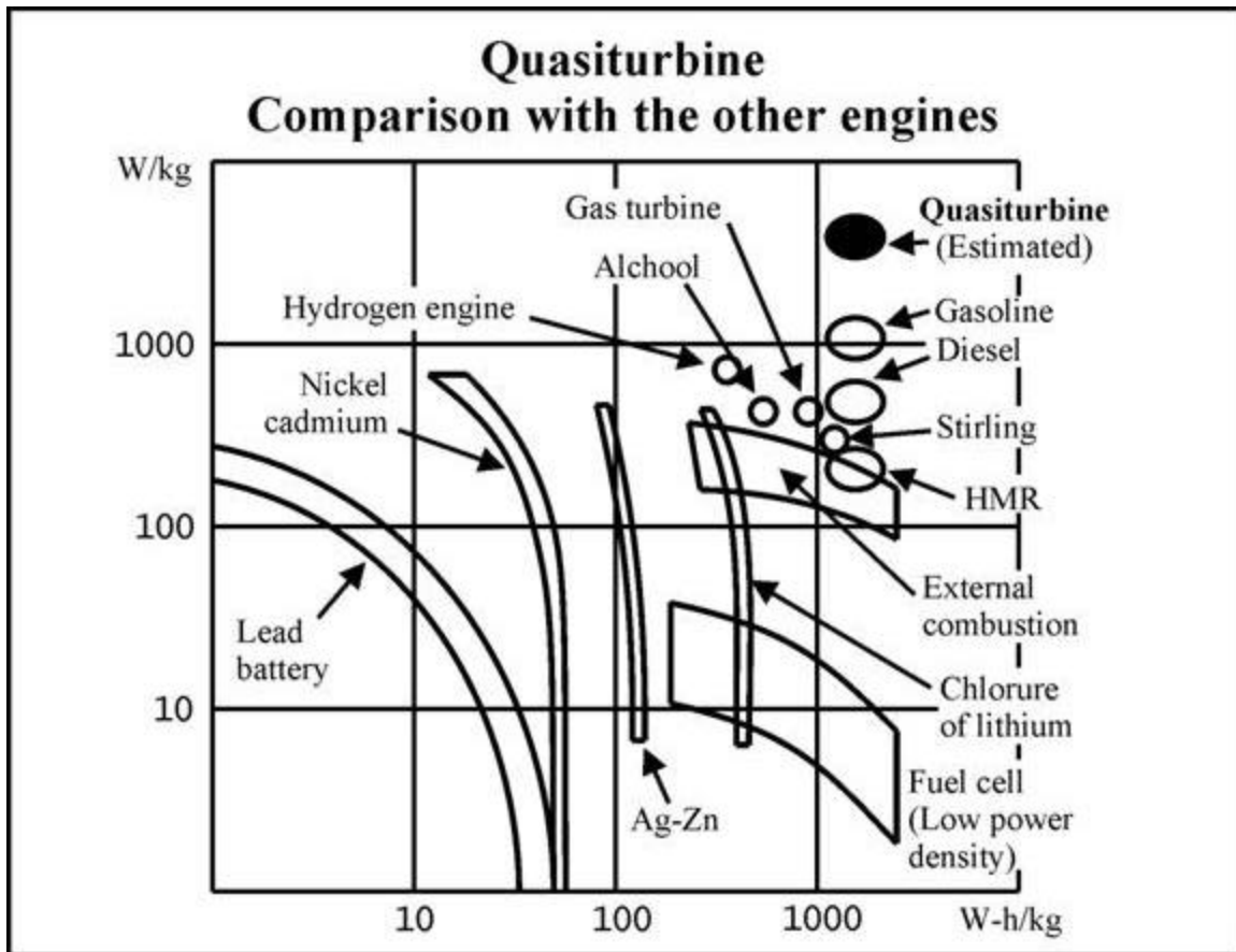
Diagramme de RAGON - Une comparaison de plusieurs moteurs de véhicule en fonction de leur densité spécifique d'énergie et densité de puissance. Notez la basse densité de puissance spécifique des piles à combustible d'hydrogène, dans le coin inférieur droit du diagramme. Référence : Romance of the engines, par Dr. Tukashi Suzuki, Éditions SAE.
